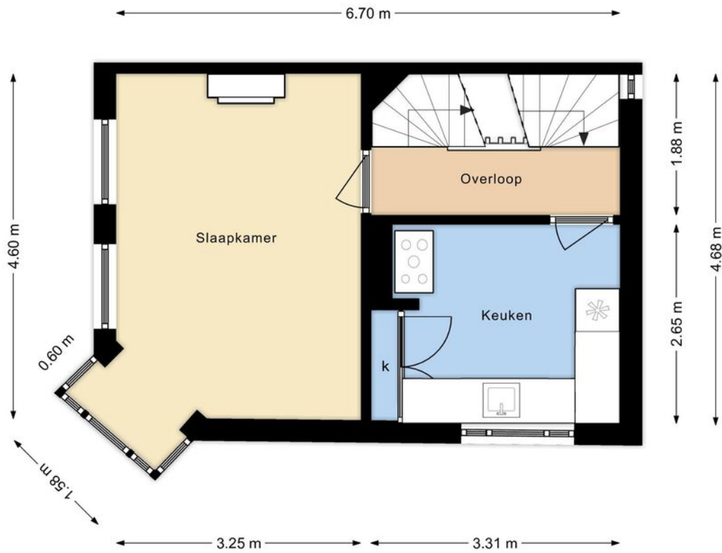
MOLENSTRAAT 24 1e Verdieping Hoogte 3.10m
