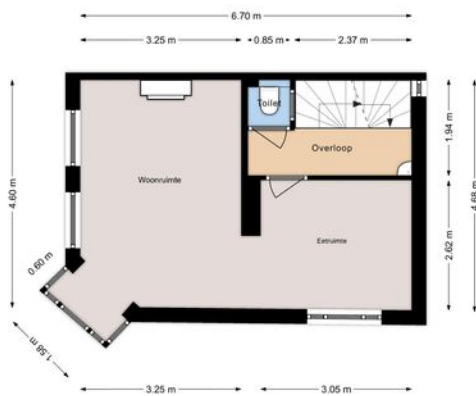
MOLENSTRAAT 24 2e Verdieping Hoogte 3.07m
