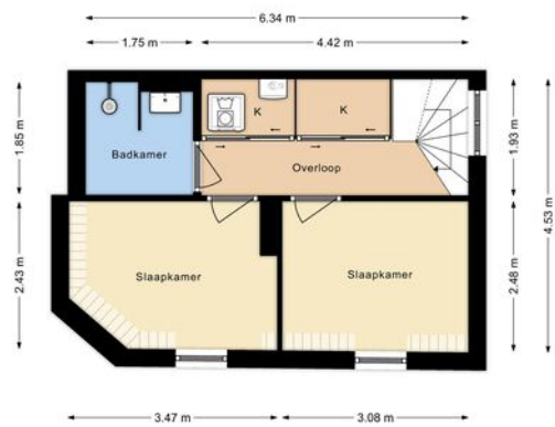
MOLENSTRAAT 24 3e Verdieping Hoogte 3.10m
